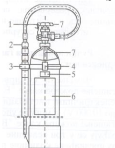
Сл. 98. Ручни апарат гашења "CO 2 "
